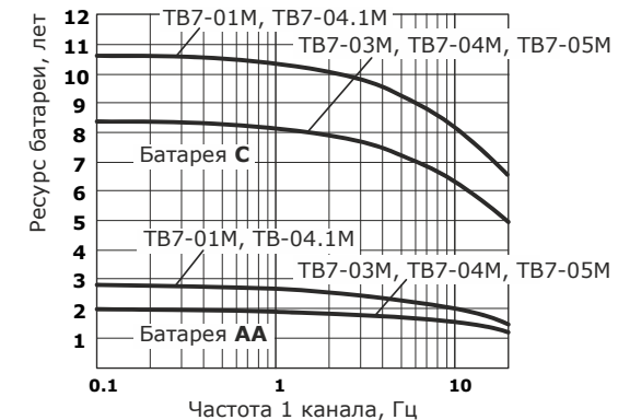
Рис. 1.1 – Ресурс батареи
