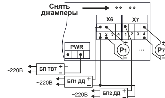
Вариант 3. Раздельное питание ТВ7 и ДД
