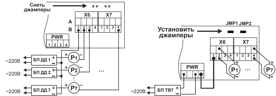
Вариант 1. Индивидуальное питание ДД
