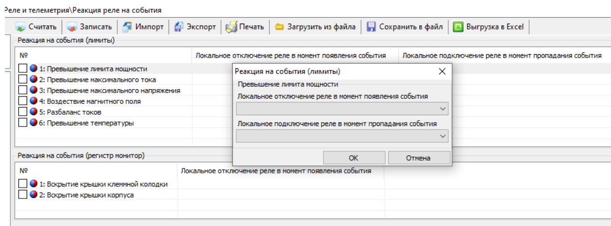
Рисунок 53 – Настройка реакций РУН на события по протоколу СПОДЭС
