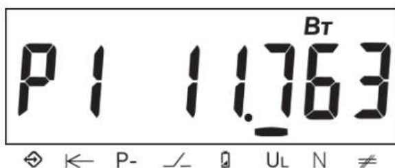
Рисунок 36 – Активная мощность по фазе.
