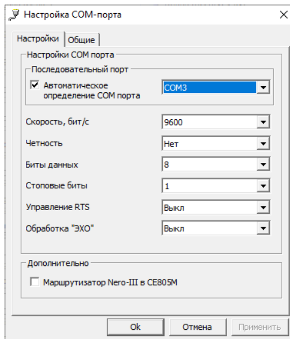
Рисунок 20 - Окно редактирования настроек канала связи «EIA-232»
