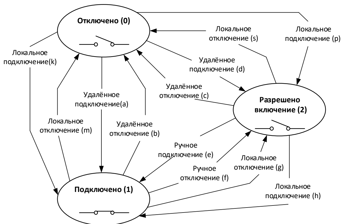
Рисунок 65 – Возможные переходы реле.
