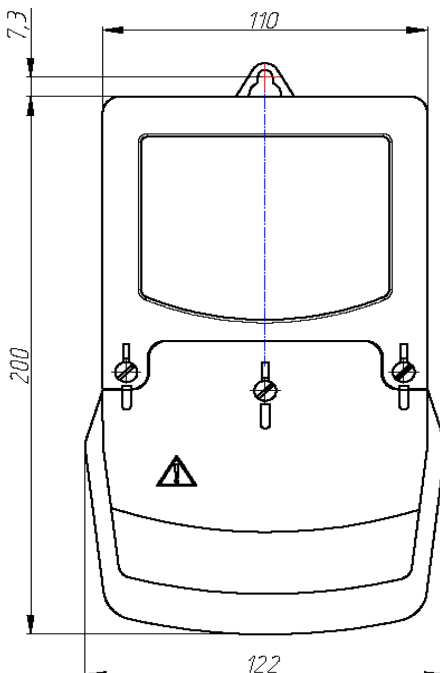
Общий вид счетчика СЕ 207 S7
