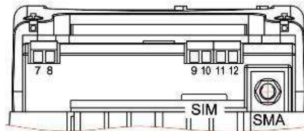
г) обозначение контактов счетчика с GSM модулем
