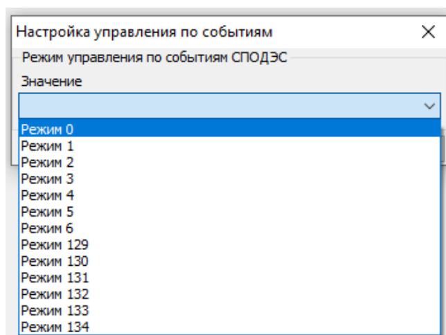
Рисунок 64 – Режимы работы реле
