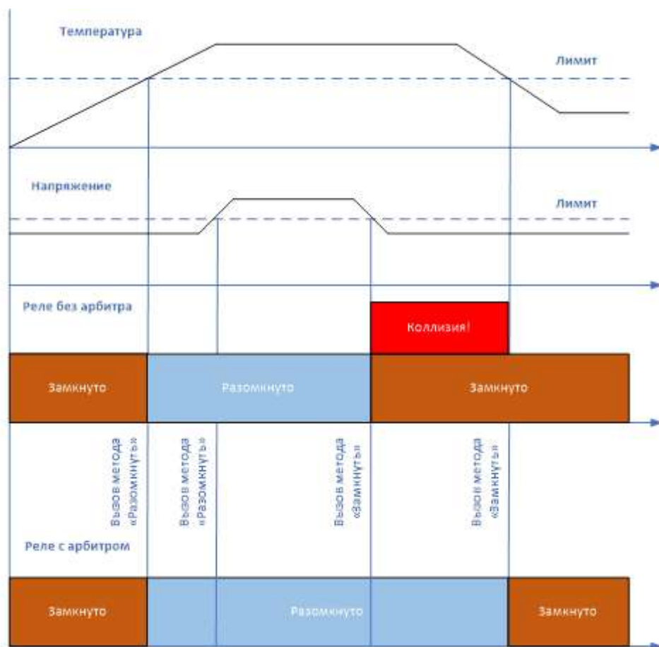
Рисунок 60 – Пример возникновения коллизии
