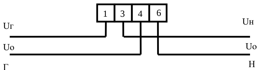
Рисунок 6 – Схема подключения СЕ 207
