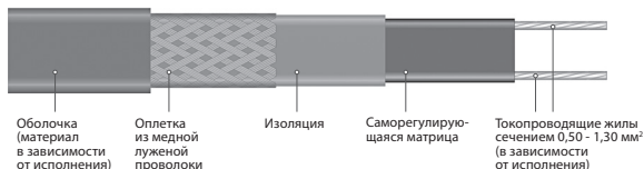
Рисунок 1. Конструкция кабеля нагревательного Freezstop
