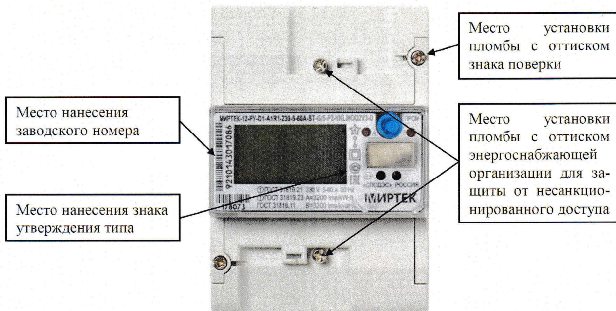
Рисунок 7 – Общий вид счетчика в корпусе типа D1
