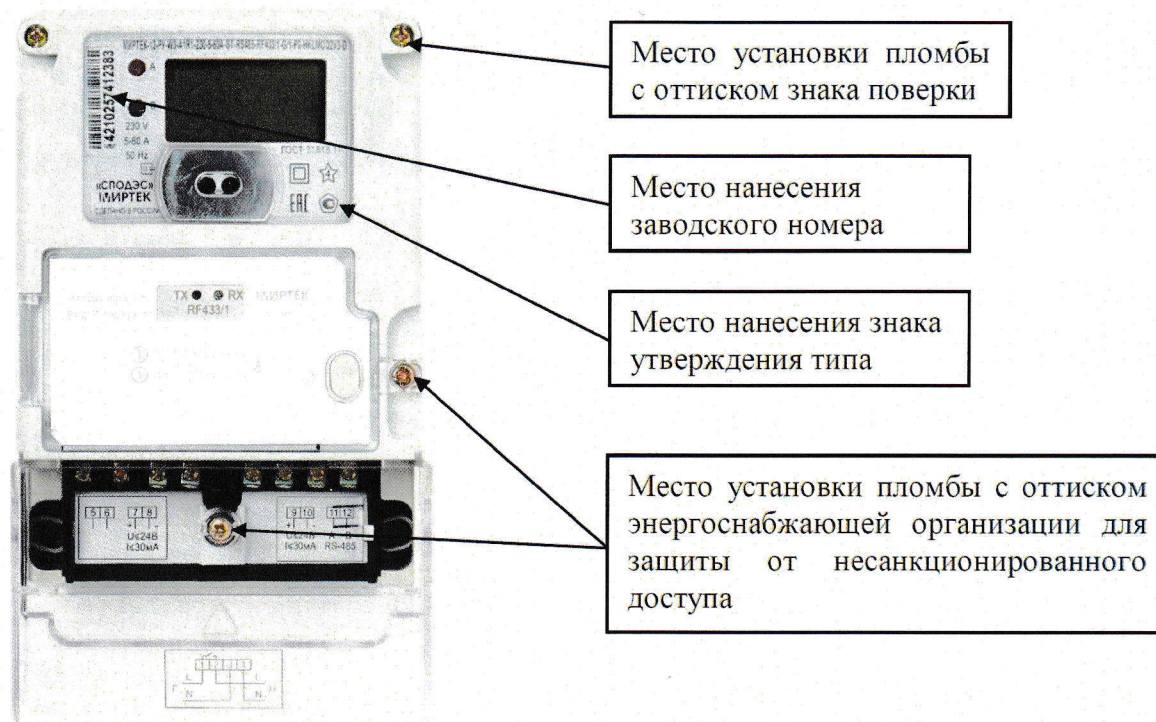
Рисунок 3 – Общий вид счетчика в корпусе типа W3
