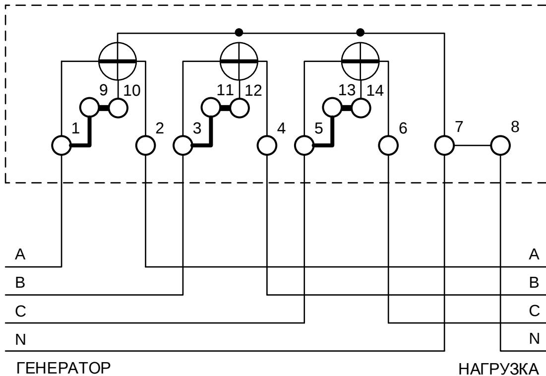
Рисунок Б.1 – Схема прямого подключения
