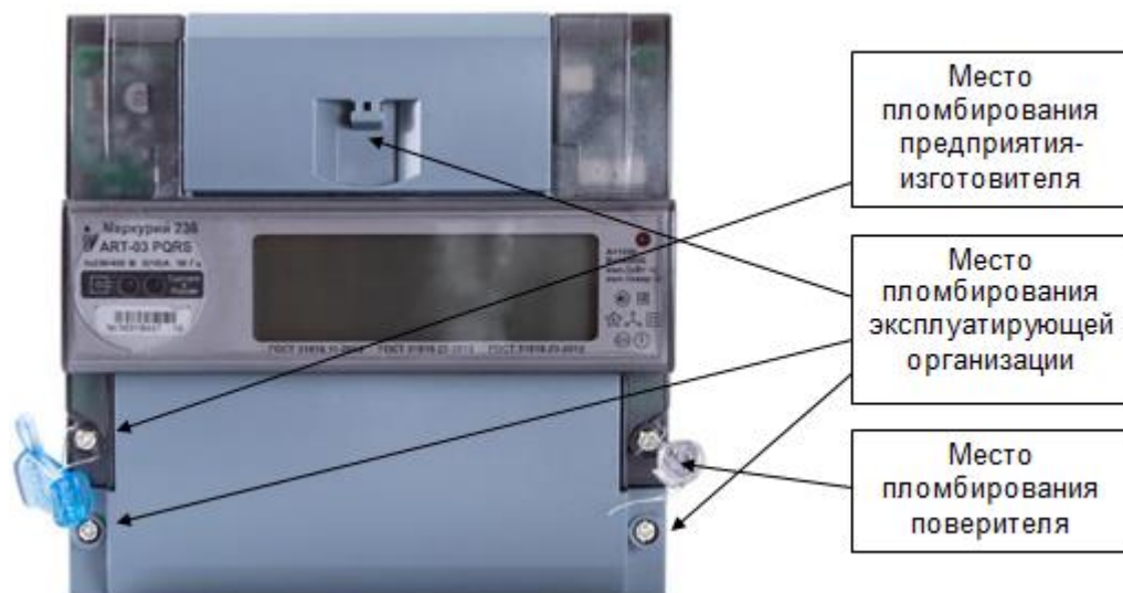
Рисунок 2.1 – Схема пломбирования
